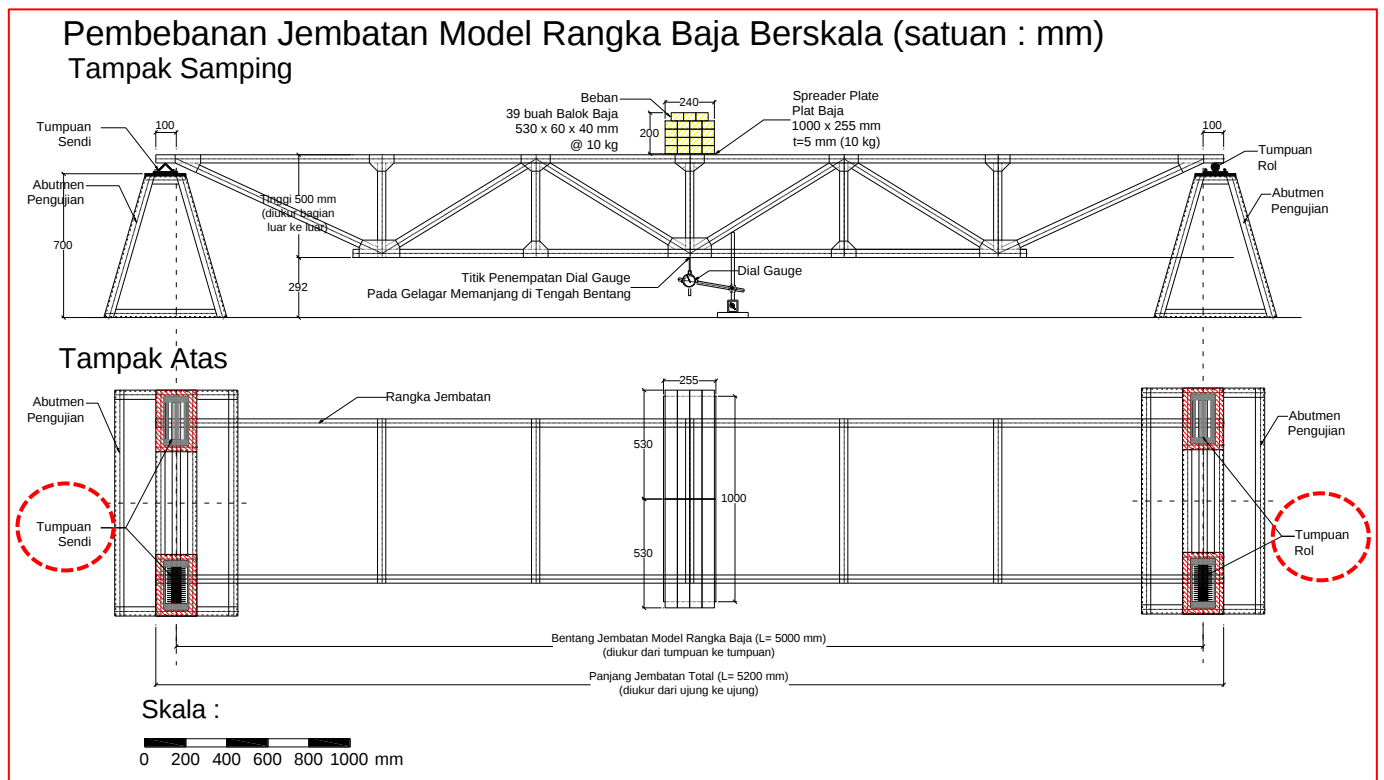
Gambar 2 Pembebanan Jembatan Model Rangka Baja
