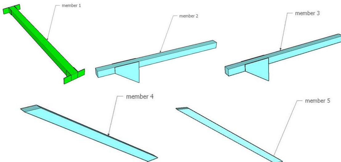
Gambar 7 Revisi dan Tambahan Contoh Pembagian Segmen Jembatan Rangka Baja
