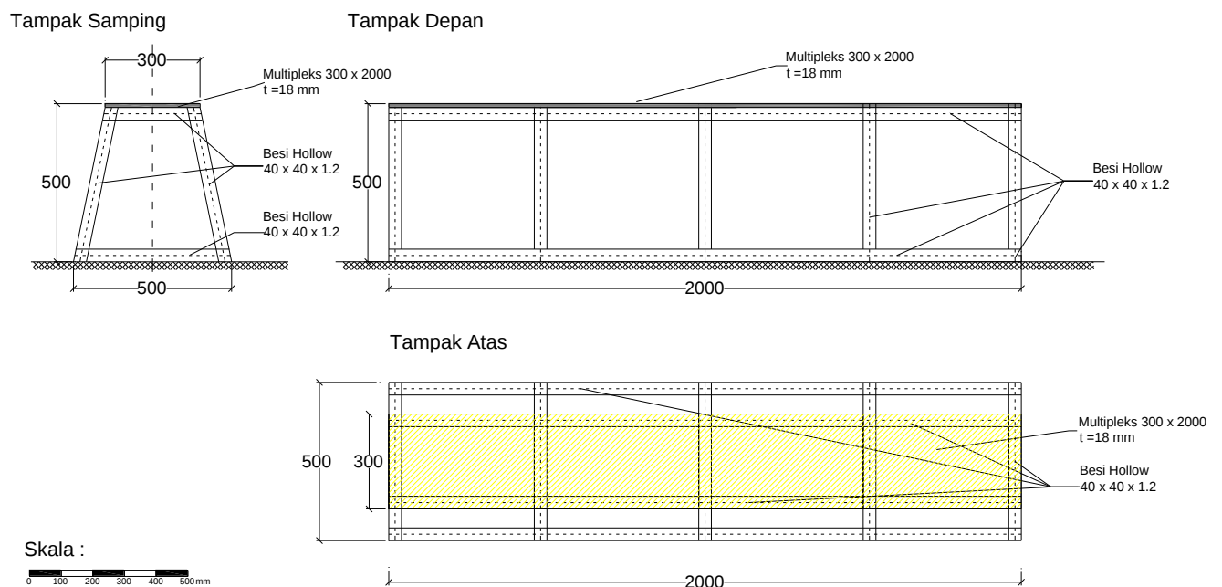
Gambar 12 Perancah untuk Perakitan Jembatan (Model Rangka Baja dan Pelengkung)
