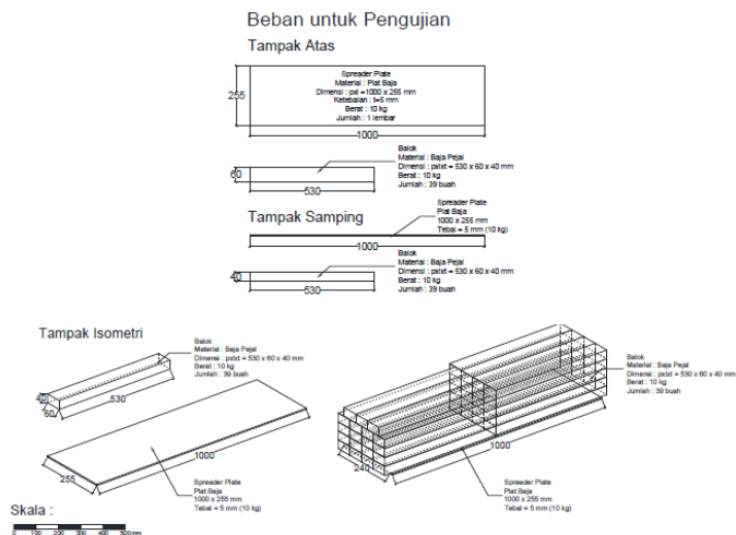
Gambar 12. Beban 400 kg Untuk Pengujian Jembatan Rangka Baja
