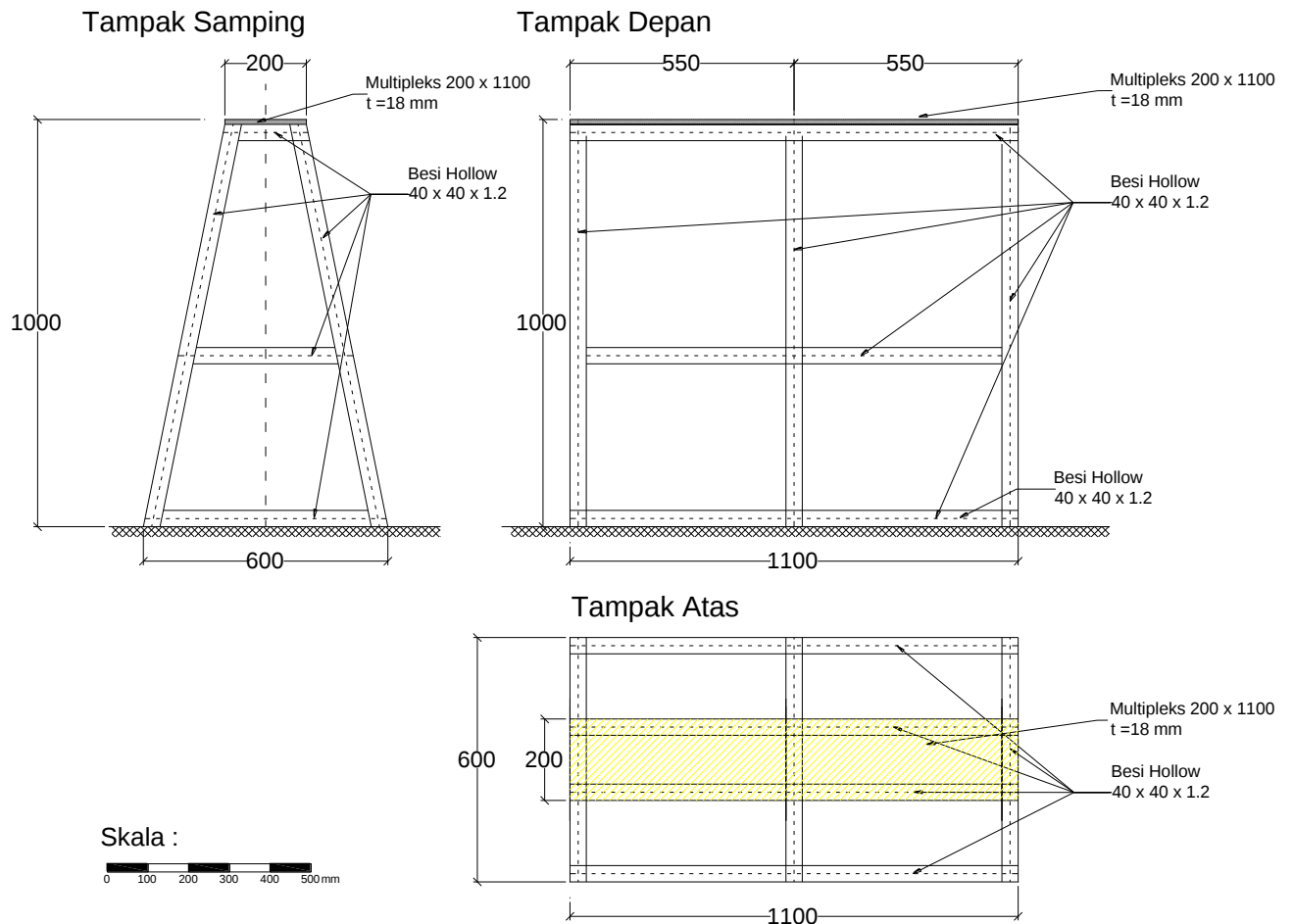
Gambar 13 Abutmen untuk Perakitan dan Display Jembatan Rangka Baja
