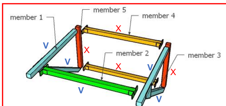
Gambar 4 Contoh Pembagian Segmen Jembatan Rangka Baja
