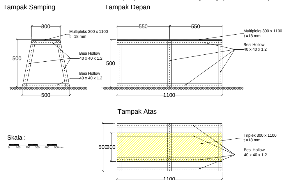
Gambar 14 Abutmen untuk Perakitan dan Display Jembatan Pelengkung
